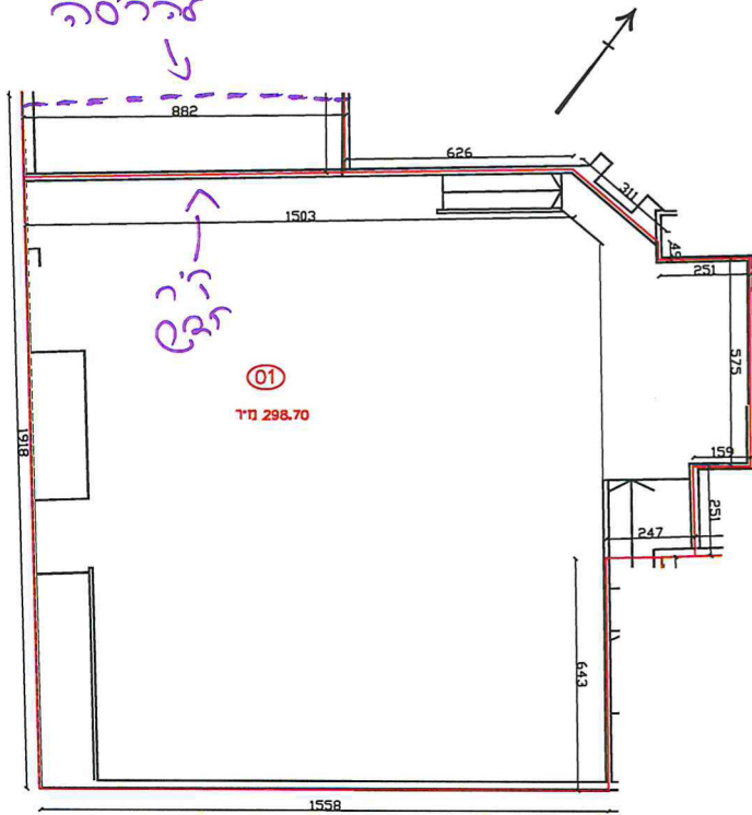
קומת קרקע
