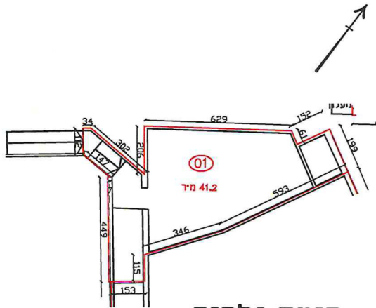
קומת גלריה
