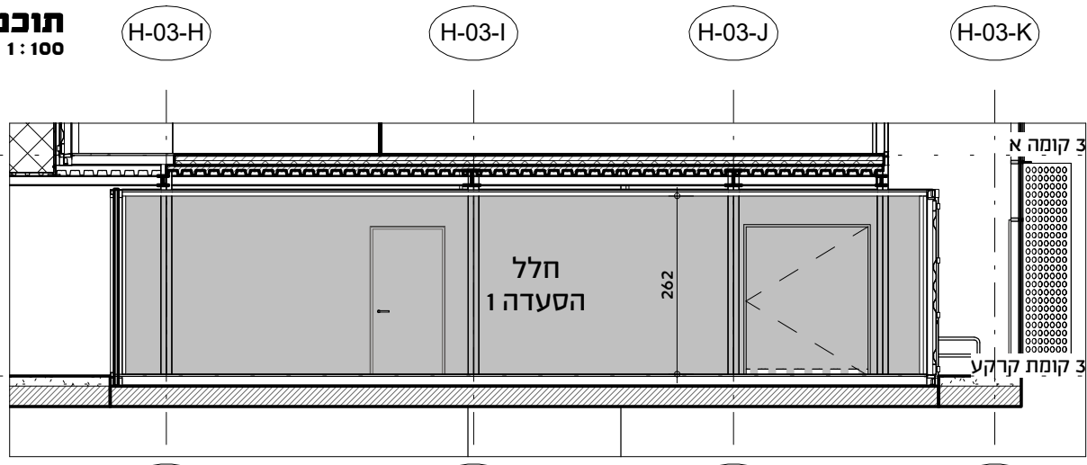
חתך 1:100
